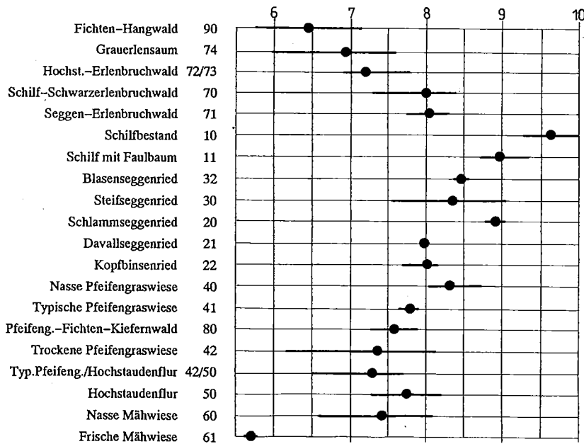
Abb. 10: Feuchtezahl der Vegetationseinheiten, hochgerechnet aus den Zeigerwerten nach ELLENBERG (1979), der dunkle Punkt kennzeichnet den Mittelwert, die Balkenbreite kennzeichnet jeweils Minimal- und Maximalwert.
